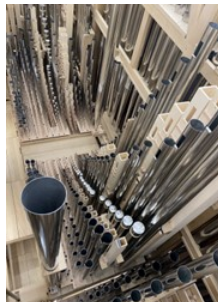
Registeraufbau Orgelwerkstatt Klais, Bonn
